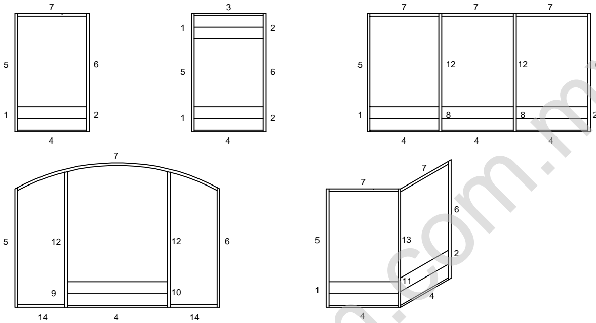
ELEVACIONES TIPO
