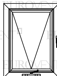
VP-50 MÍNIMO 0.60 x 0.60 MÁXIMO 0.90 x 1.80
